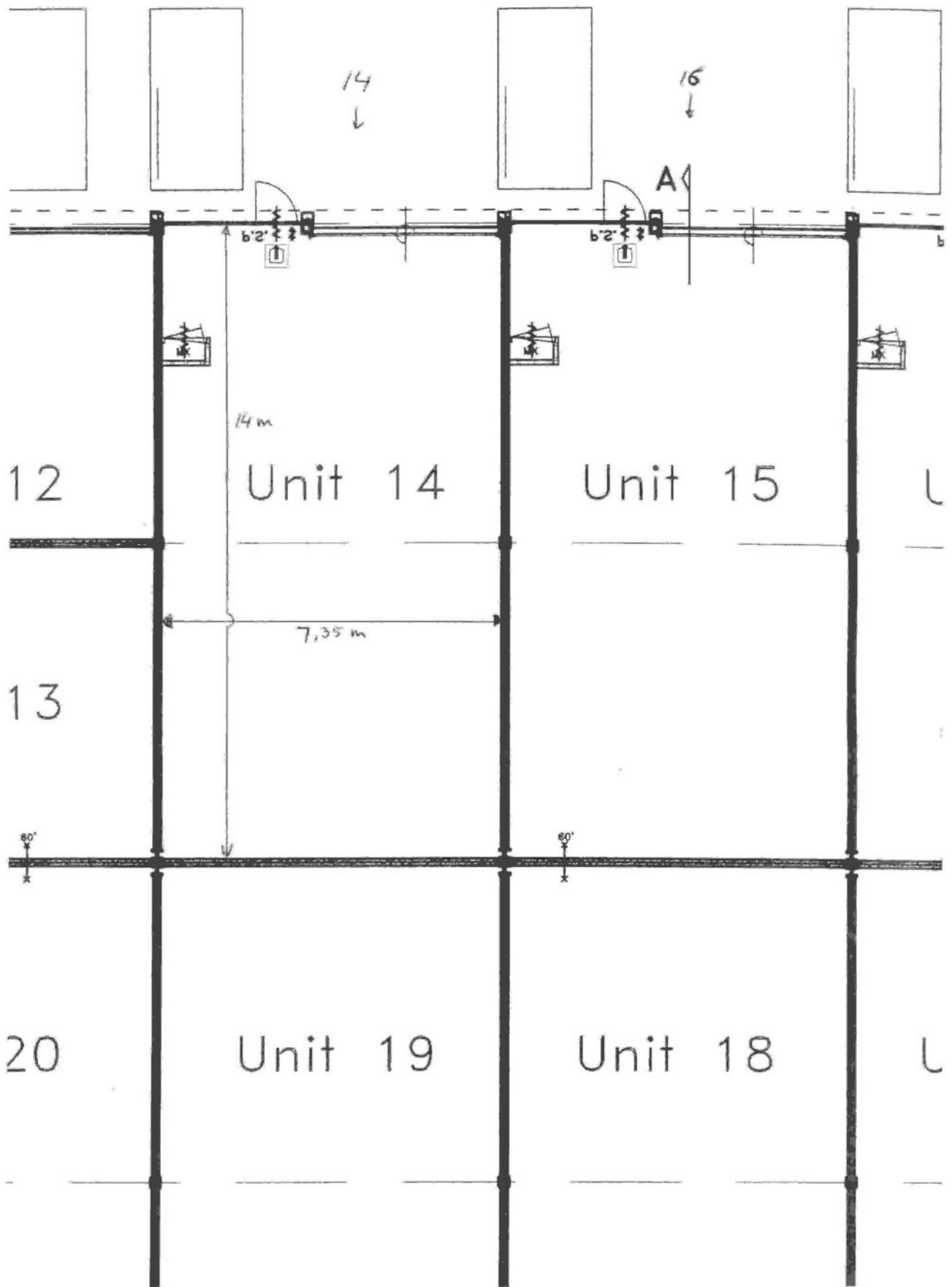
PLATTEGROND
