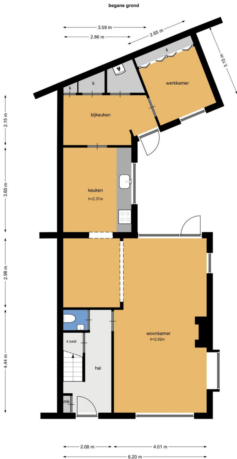
PLATTEGROND BEGANE GROND
