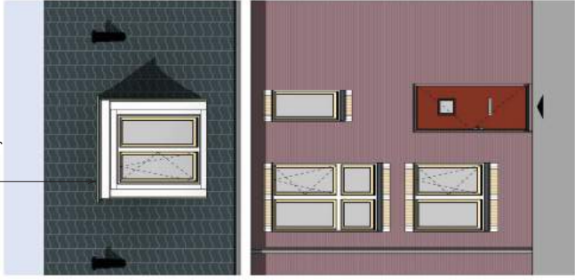
Voorgevel Blok 3: Nr. 108, 109, 110 en 111
